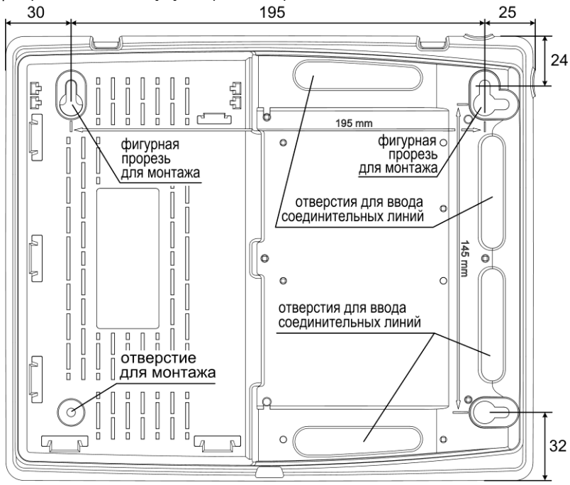
Рис.3 Задняя стенка прибора. Присоединительные размеры
